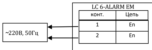
Рис.1. Схема подключения.
